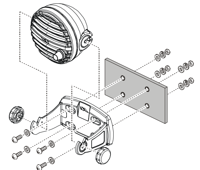
Figure 2 (Wall Mount)
