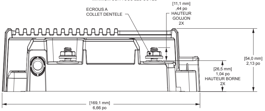
VUE AVEC COUVERCLE DEPOSE
