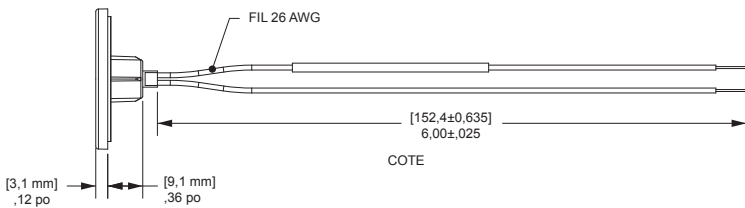
VUE AVEC COUVERCLE DEPOSE
